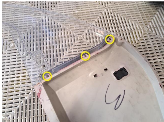
Irrota sivuikkunan sivupaneelissa kiinni pitävät kiinnitysruuvit (ristipäämeisseli ph2).
