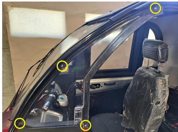
Irrota sivuikkunan kiinnitysruuvit (ristipäämeisseli ph2).
